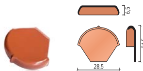
zamknięcie końcowe kalenicy nr 11
