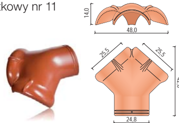
trójkąt końcowy nr 11
